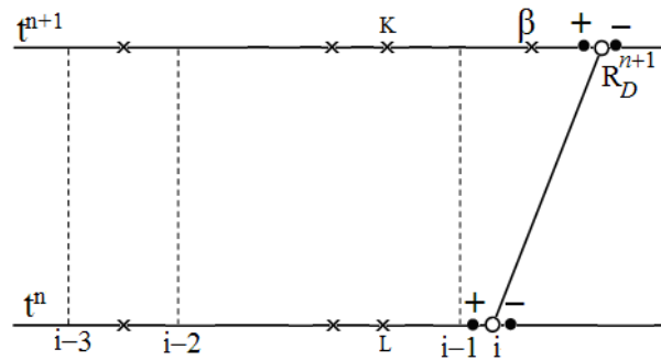
Рис.5. Расчет \beta -интервала при выходе разрыва из целой точки
