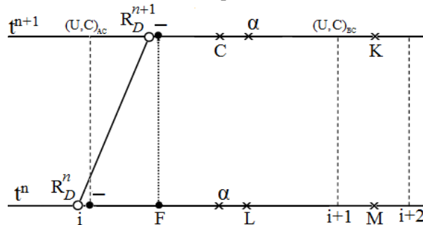
Рис.3. Расчет «альфа» величин
