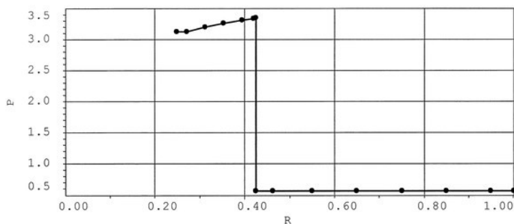
Рис.9 – Распределение давления в системе на момент времени t= 0.2557
