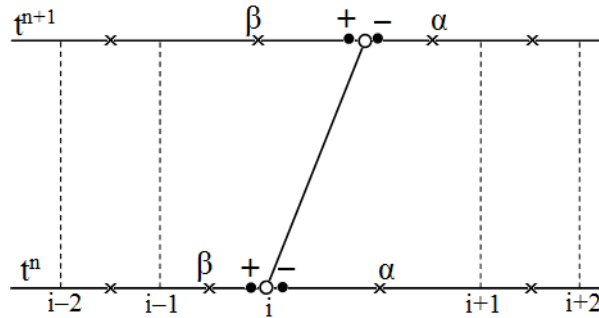
Рис. 1. Шаблон расчета особого интервала
