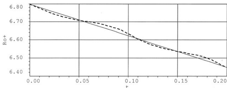
Рис. 8 – Зависимости плотности за фронтом от времени.
