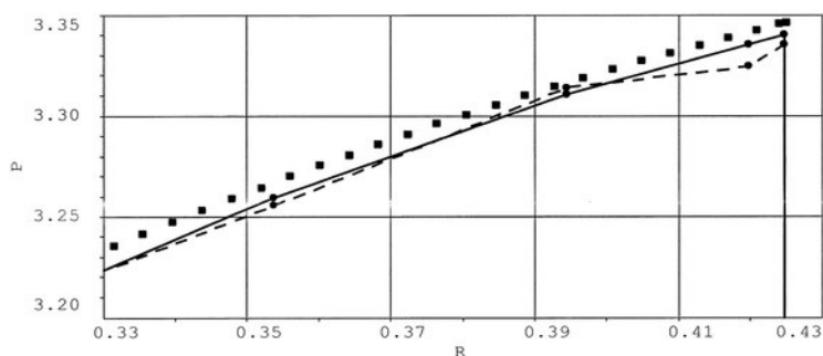
Рис.10 – Распределение давления в области за фронтом на момент времени t= 0.2557 .
