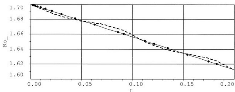
Рис. 7 – Зависимости плотности перед фронтом от времени.
