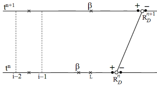
Рис.4. Расчет величин в интервале за фронтом
